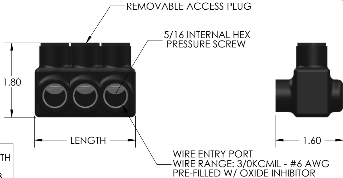
IPL3/0-3 SHOWN
